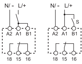
Esquema de conexión (sin señal de mando)
